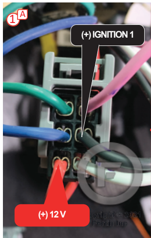
① At ICU, junction block-dash fuse box Au ICU, boîte à fusibles bloc de jonction du tableau de bord
