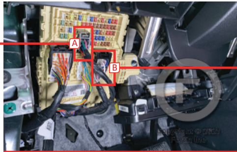
① At ICU, junction block-dash fuse box Au ICU, boîte à fusibles bloc de jonction du tableau de bord
