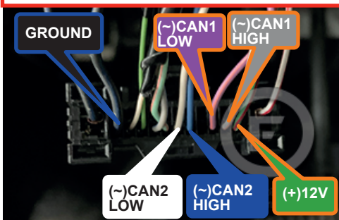
③ Gateway module, Behind OBD-II connector Module Passerelle réseau, Derrière le connecteur OBD-II
