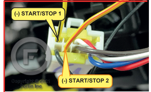
④ At Push-to-start button Au bouton de démarrage
