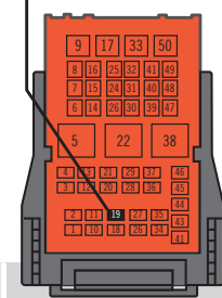
① Back view - 50-Pin Red Connector in the driver's side kick panel Vue de dos Connecteur Rouge de 50-Pins Panneau latéral côté conducteur
