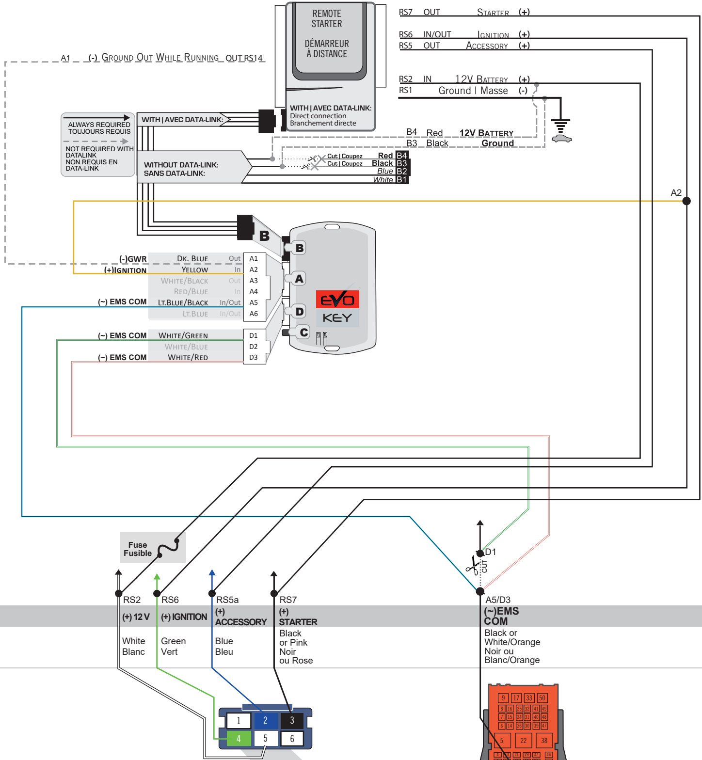
② Back view - Blue 6-pin connector, at ignition connector. Vue de dos - Connecteur Bleu, 6-pins, au connecteur d'ignition.
