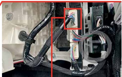
④ At certification ECU, Behind glove box Au ECU certification, Derrière la boîte à fusibles
