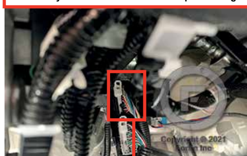
② Hybrid ECU located above gas pedal. ECU Hybride situé au-dessus de la pédale de gaz.
