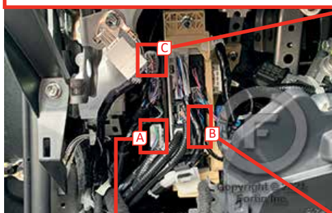
① At junction connector, Driver's side Au connecteur de jonction, Côté conducteur
