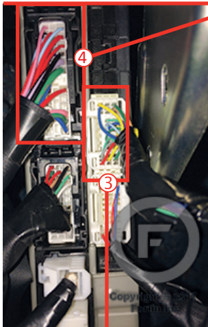
③ ④ Left side of driver's dash Gauche de la tableau de bord côté conducteur
