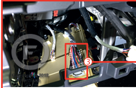
③ Rear of the Fusebox/Smart Junction Dos de la boîte à fusibles/Smart Junction
