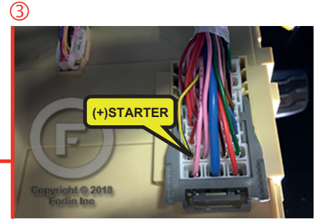
③ Rear of the Fusebox/Smart Junction Dos de la boîte à fusibles/Smart Junction
