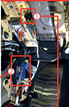
① ② Fusebox / Smart Junction Boîte à fusibles/Smart Junction
