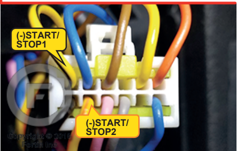
④ Start Stop Button Switch Commutateur du bouton démarrage
