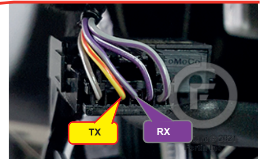
① Immobiliser immobilisateur RX and TX of the module RX et TX du module
