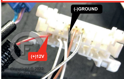
① OBDII connector Connecteur OBDII
