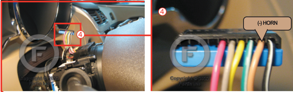
④ At steering column À la colonne de direction
