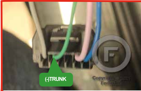
③ At trunk Switch Au commutateur de la valise
