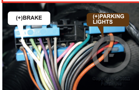
2 At Driver kick panel Au Panneau latéral côté conducteur
