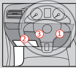
① Back view - Blue 6-pin connector, at ignition connector. Vue de dos - Connecteur Bleu, 6-pins, au connecteur d'ignition.
