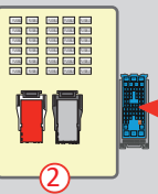
Back view Blue 71-pin connector Right of the Fusebox. Vue de dos Connecteur Bleu de 71 pins À droite de la boîte à fusibles
