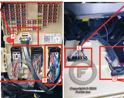
② Fusebox / Smart Junction Box Boîte à fusibles/Smart Junction
