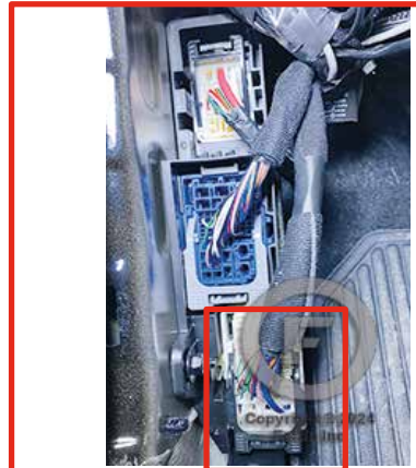
① In the driver's side kick panel Panneau latéral côté conducteur
