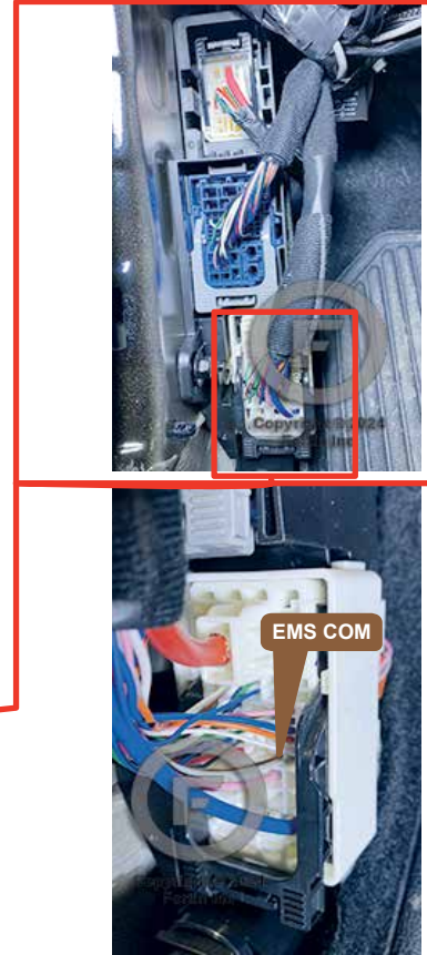
① In the driver's side kick panel Panneau latéral côté conducteur
