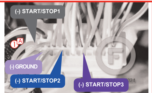
1 ECU, behind glove box ECU, derrière le coffre à gant
