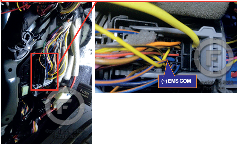
① Driver kick Panel Panneau latéral côté chauffeur
