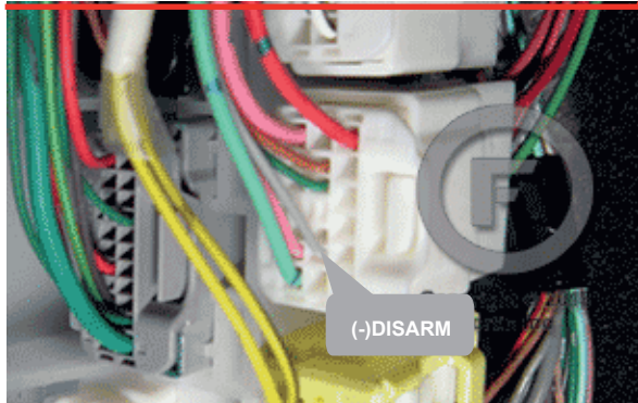
⑤ Driver's kick panel Panneau latérale côté conducteur
