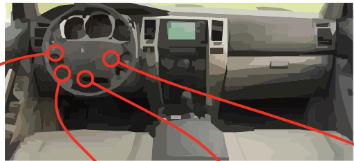
OBD-II connector Connecteur OBD-II
