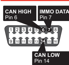
OBD-II connector Connecteur OBD-II
