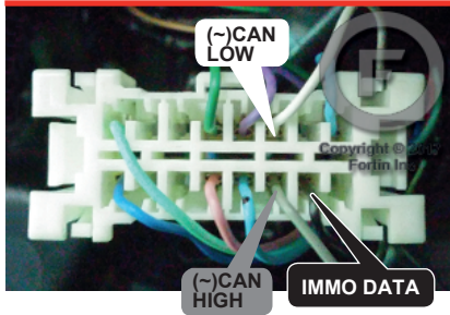
② OBD-II connector Connecteur OBD-II
