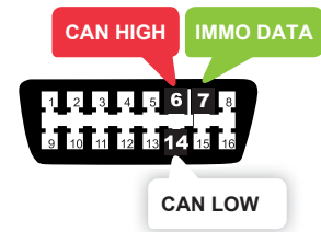
② OBD-II connector Connecteur OBD-II
