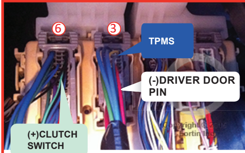
③ ⑥ Fuse box Boîte à fusibles
