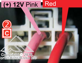
(+) 12V Pink
