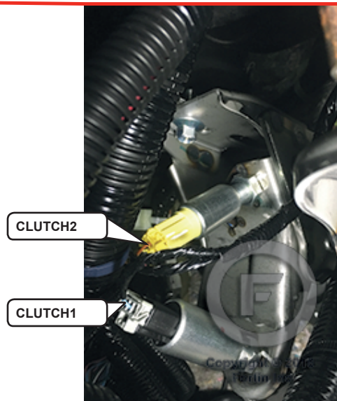
⑥ ⑦ Clutch switch Commutateur d'embrayage
