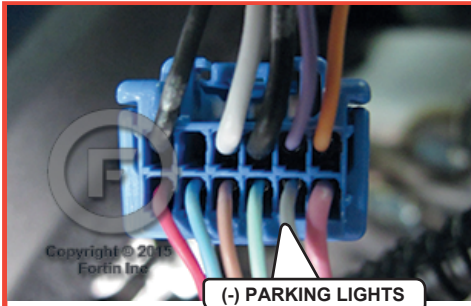
④ Parking Light Switch Commutateur des feux de stationnement.
