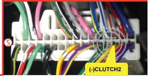
⑤ Under steering column, START-STOP unit. Sous la colonne de direction, unité DÉMARRAGE.
