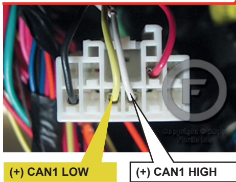
④ Fuse panel (back) Au dos de la Boîte à fusibles
