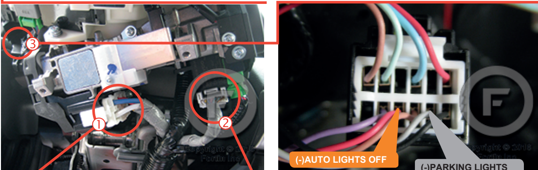
Ignition key barrel Barillet d'ignition
