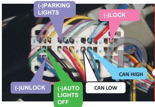
③ ④ ⑤ MAIN BODY ECU LEFT SIDE OF THE DASH CÔTÉ GAUCHE DU TABLEAU DE BORD
