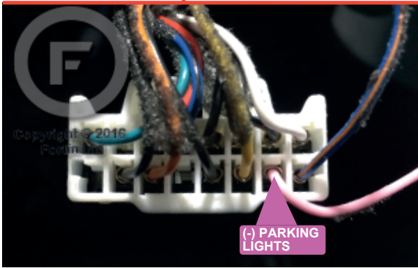
2 Driver kick panel Panneau latéral côté conducteur
