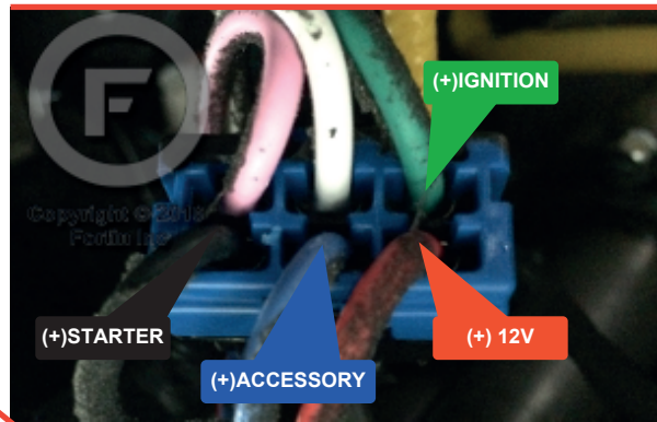
1 Ignition connector Connecteur d'ignition
