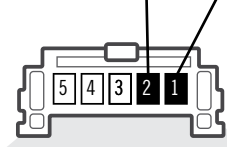
① Back view - 5-Pin - White Connector - OEM remote starter connector, behind glove box. Vue de dos - 5-Pins - Connecteur Blanc - Connecteur de démarrage à distance d'origine, derrière le coffre à gants.
