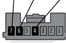
② Back view 7-Pin Black Connector Steering Lock Connector Vue de dos Connecteur Noir 7-Pins Connecteur Steering Lock
