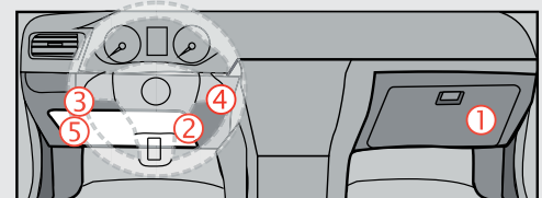
① Back view - 5-Pin - White Connector - OEM remote starter connector, behind glove box. Vue de dos - 5-Pins - Connecteur Blanc - Connecteur de démarrage à distance d'origine, derrière le coffre à gants.
