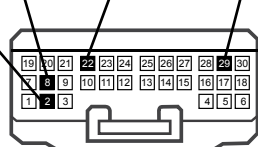
③ Back view - 30-Pin - White Connector Vue de dos - 30-Pins - Connecteur Blanc
