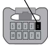
④ Back view 10-Pin Black Connector Push-to-start button Vue de dos Connecteur 10-Pins Noir Bouton démarrage
