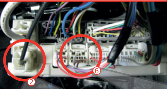
②⑥ ECM Driver Kick Panel ECM ECM Panneau latéral côté chauffeur
