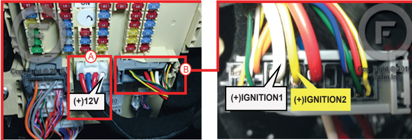
③ Front of fuse box Devant de la boîte à fusible
