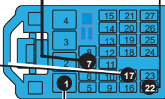
② Back view, 27-Pin Blue connector, at BCM. Vue de dos, connecteur Bleu 27-Pins, au BCM.
