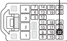
① Back view, 26-Pin White connector, at BCM. Vue de dos, connecteur Blanc 26-Pins, au BCM.
