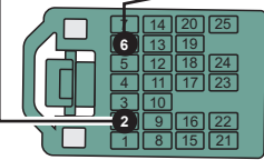
③ Back view, 25-Pin Green connector, at BCM. Vue de dos, connecteur Vert 25-Pins, au BCM.
