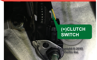
⑤ Clutch switch Commutateur d'embrayage
