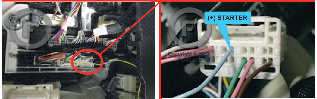
④ Certification ECU, behind glove box Certification ECU, derrière le coffre à gants
