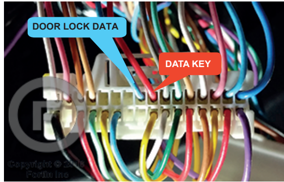
① Under steering column, START-STOP unit Sous la colonne de direction, unité DEMARRAGE
