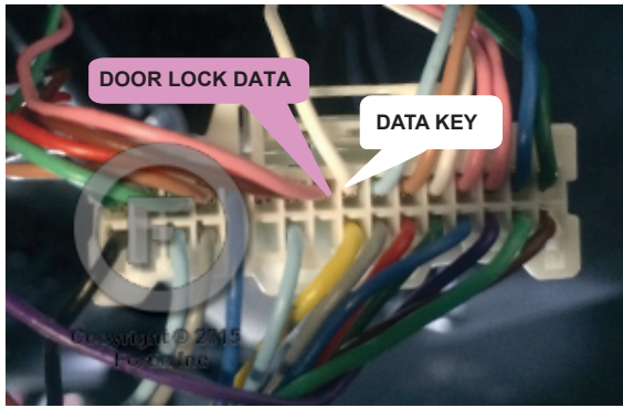
① Under steering column, START-STOP unit Sous la colonne de direction, unité DÉMARRAGE
