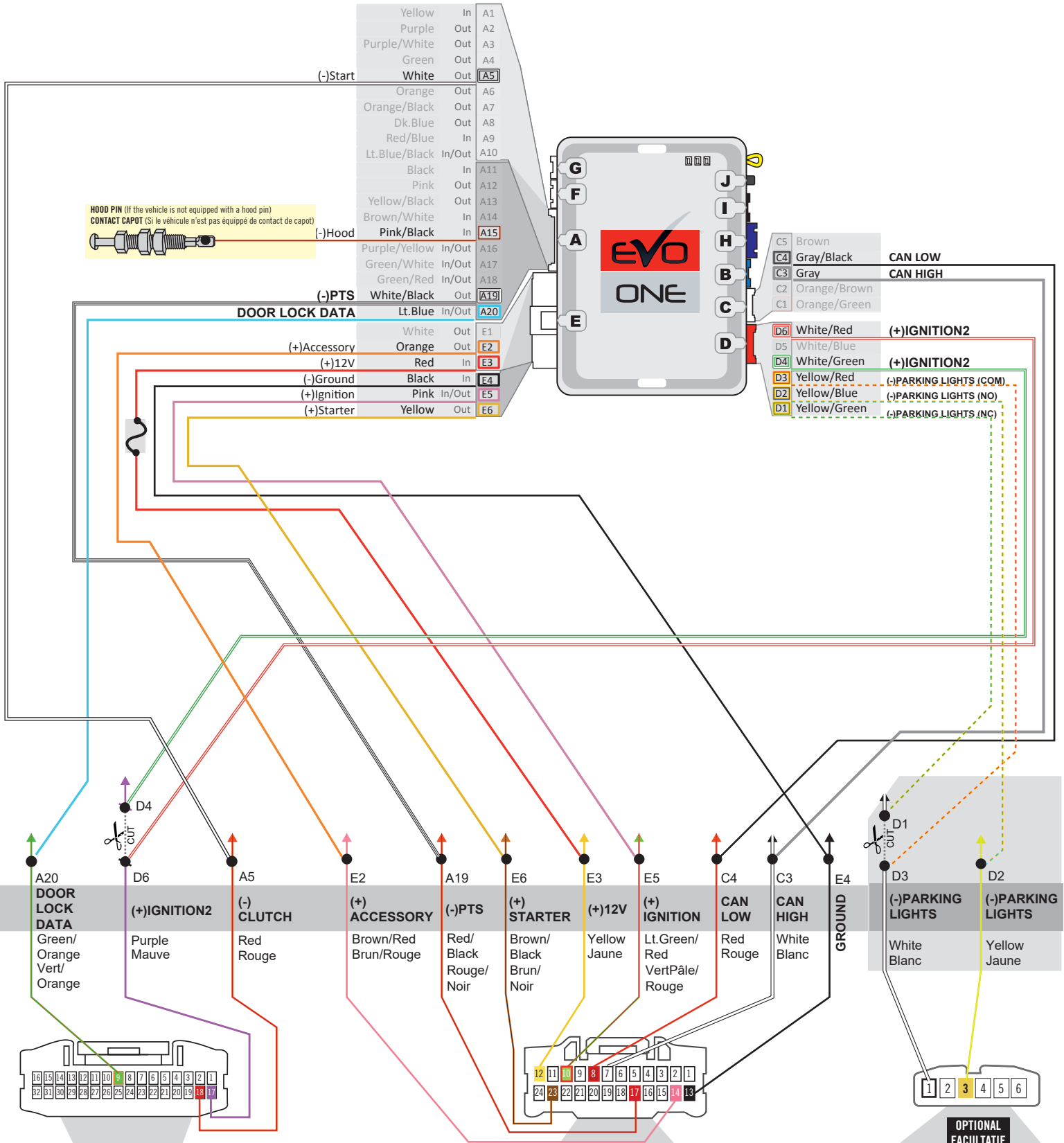
② Back view. 32-pin White connector. Under steering column, START-STOP unit. Vue de dos. Connecteur Blanc 32-pins. Sous la colonne de direction, unité DÉMARRAGE.
