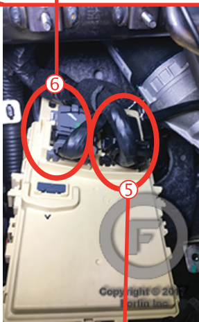
⑤⑥ Back of Fuse Box Au dos de la boîte à fusibles
