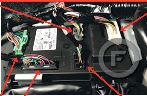
BCM located passenger kick panel. BCM Situé au panneau latérale côté passager.
