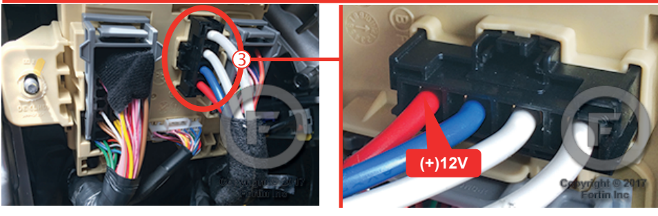
③ In the front of the fuse box Au devant de la Boîte à fusibles
