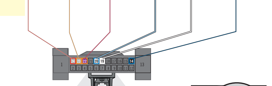
① Gateway module, Behind OBD-II connector - located at dash board driver's side - Back view, 24-pin black connector. Module Passerelle réseau, Derrière le connecteur OBD-II situé dans le tableau de bord, côté conducteur. Vue de dos, connecteur Noir de 24-pin.
