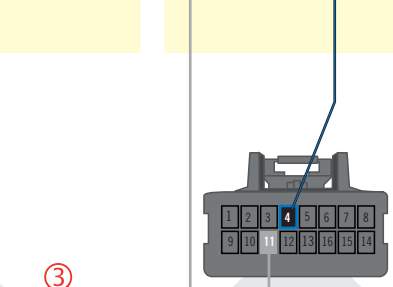
② Back view Parking Lights switch 14-pin Black Connector Vue de dos Commutateur des feux de stationnement Connector Noir 14-pins
