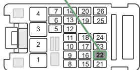
① Back view 26-Pin White Connector At BCM Vue de dos Connecteur Blanc de 26-Pins Au BCM
