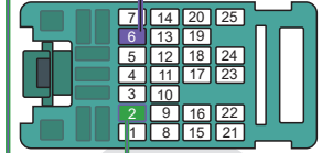
③ Back view 25-Pin Green Connector At BCM Vue de dos Connecteur Vert de 25-Pins Au BCM
