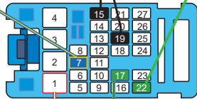
② Back view 27-Pin Blue Connector At BCM Vue de dos Connecteur Bleu de 27-Pins Au BCM
