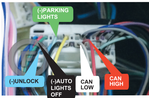
② MAIN BODY ECU LEFT SIDE OF THE DASH CÔTÉ GAUCHE DU TABLEAU DE BORD
