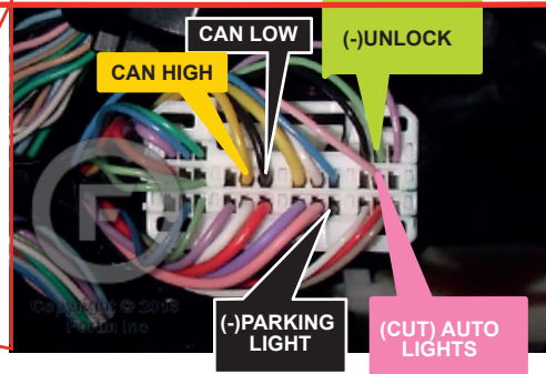
② MAIN BODY ECU / Driver's side dash. MAIN BODY ECU / tableau de bord côté conducteur.
