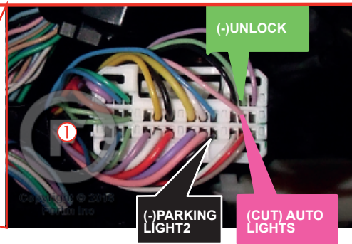
① MAIN BODY ECU / Driver's side dash. MAIN BODY ECU / tableau de bord côté conducteur.
