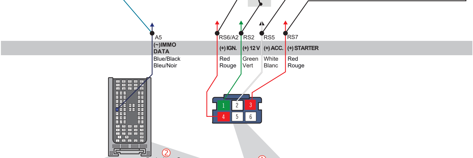
② Back view - Grey 82-pin connector - In the driver's side kick panel Vue de dos - Connecteur Gris de 82-pins - Panneau latéral côté conducteur
