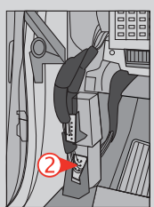
② Back view - Grey 82-pin connector - In the driver's side kick panel Vue de dos - Connecteur Gris de 82-pins - Panneau latéral côté conducteur
