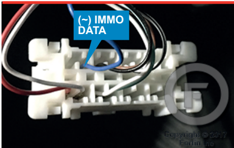
④ OBDII Connector Connecteur OBDII
