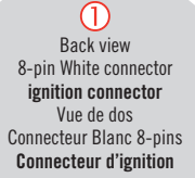
① Back view 8-pin White connector ignition connector Connecteur Blanc 8-pins Connecteur d'ignition
