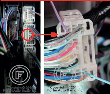
② Body ECU, on dash fuse box Body ECU, situé au-dessus de la Boîte à fusibles
