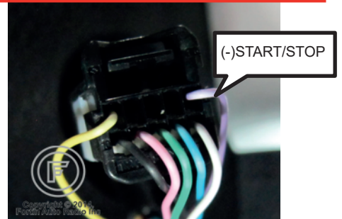
③ Push-to-start button Au bouton de démarrage
